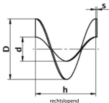
rechtslopend
